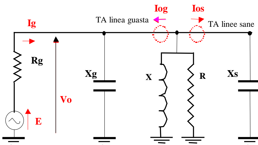
Figura 2- Circuito di riferimento per rete a NC
